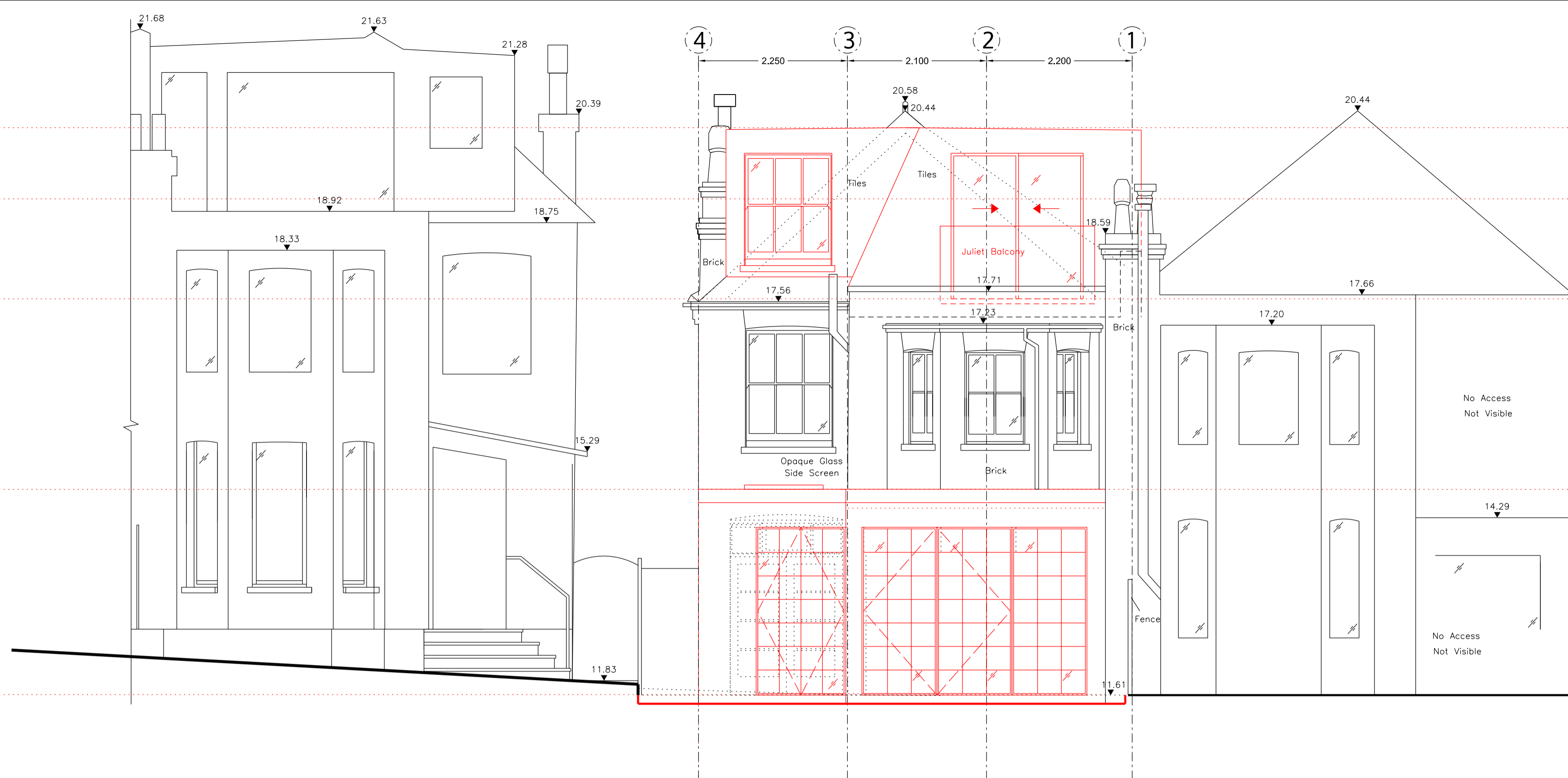
E3 REAR ELEVATION
