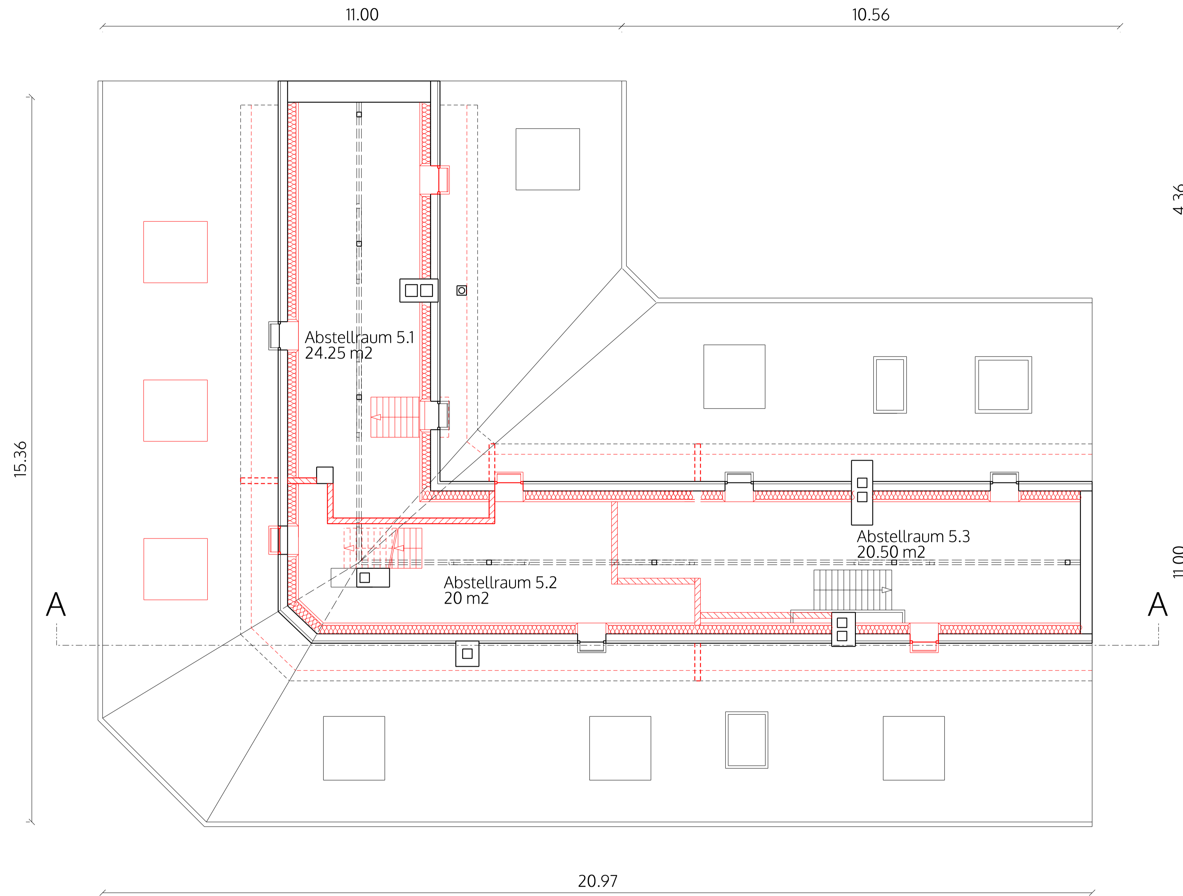
5. Obergeschoss _ plan
