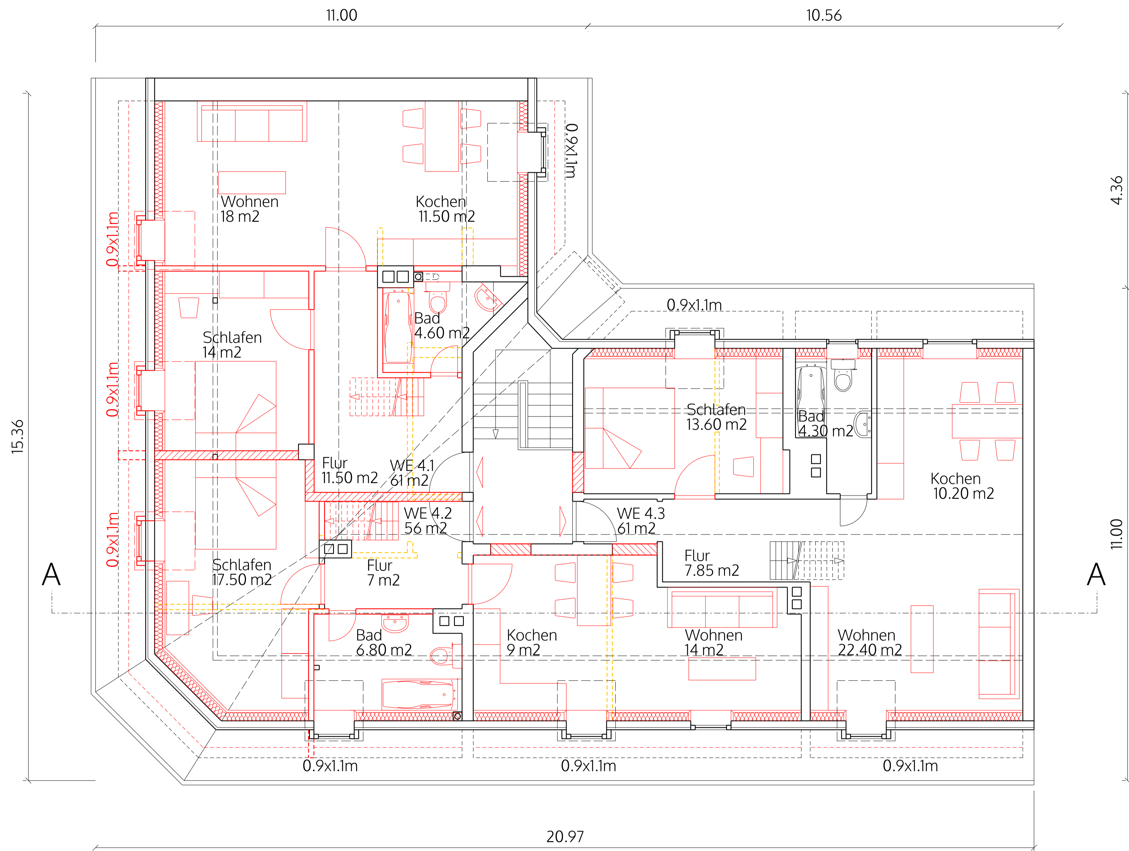
4. Obergeschoss _ plan
