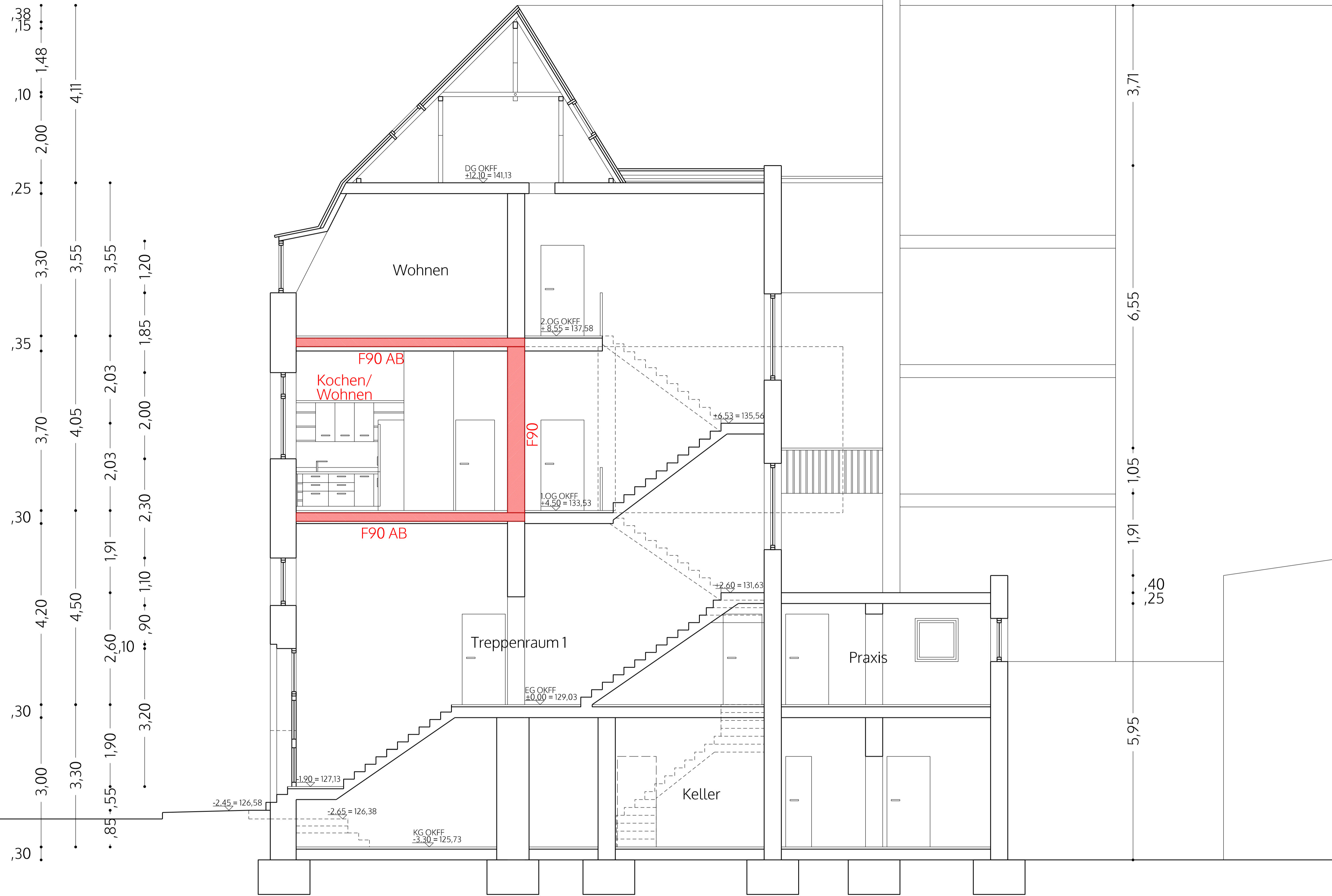
Schnitt A - A
