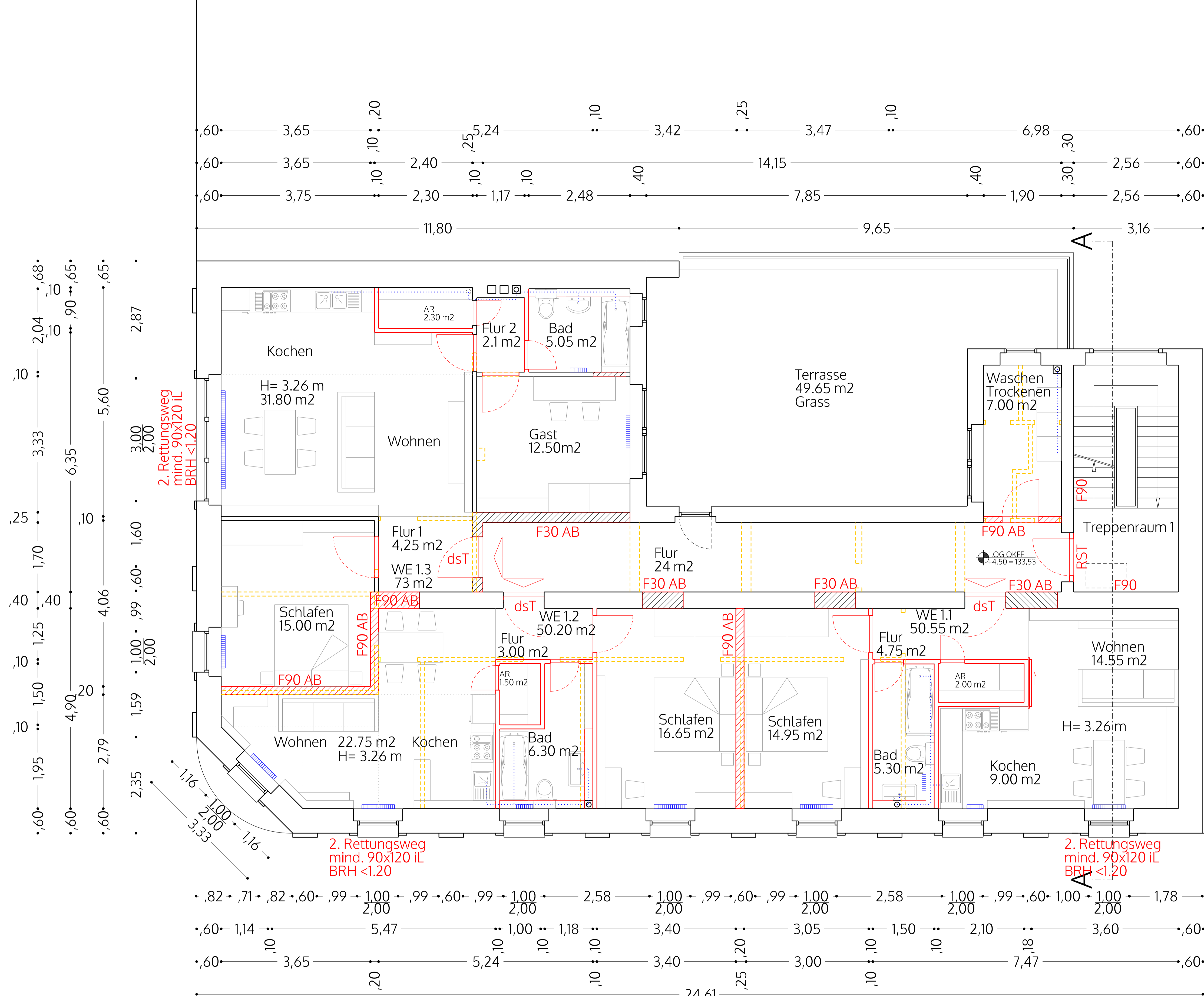
1. Obergeschoss _ plan
